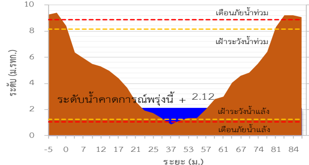
TC220605 สะพานตำรัง
