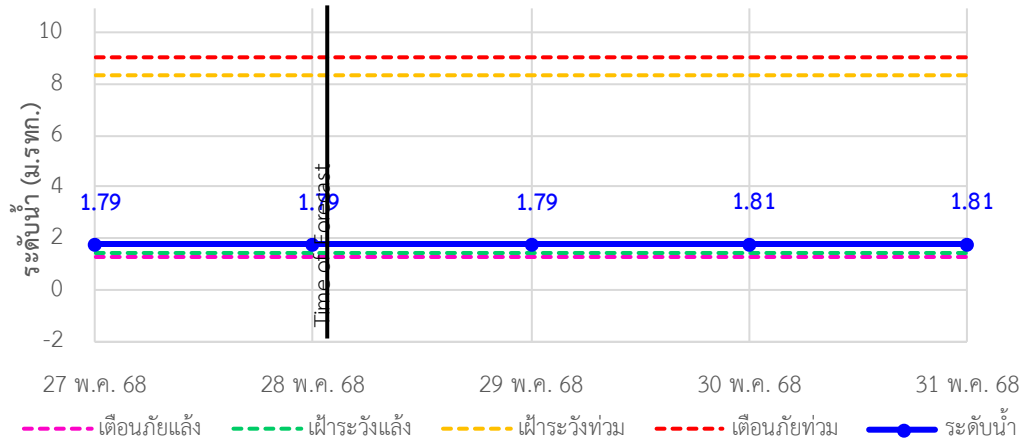
TC220512 สะพานบ้านท่าคลอง ตำบลทับปรึง อำเภอมืองกระบี่ จังหวัดกระบี่
