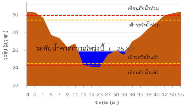
TC221202 สะพานควนโดนโน
